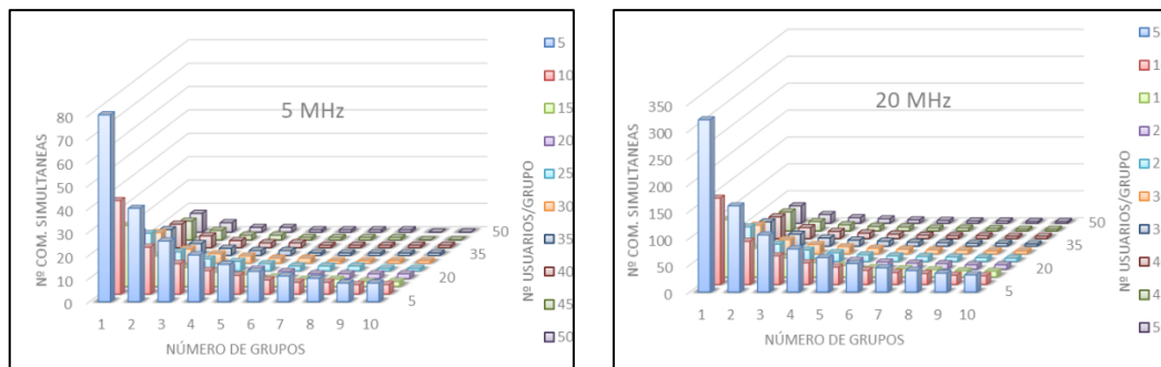
Figura 4 Evolución del número de comunicaciones simultáneas según el número y tamaño de los grupos en una misma celda Unicast (Fuente: Elaboración Propia)
