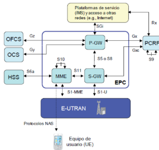
Figura 1 Arquitectura básica de la red LTE (Fuente: [8])
